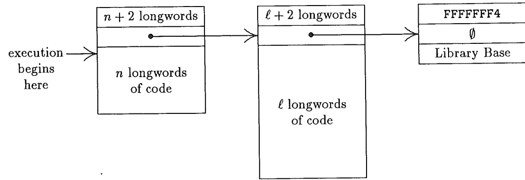
Fig. 2—The AmigaDOS SegList
